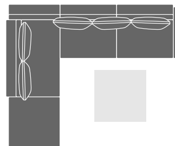
MLR.COMB3.L/R L345 B280 H70
