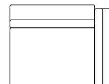
MLR.110.04.R/L L140 B105 H70
